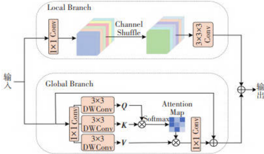
图 4.5 CAFm 结构图（待修改）
