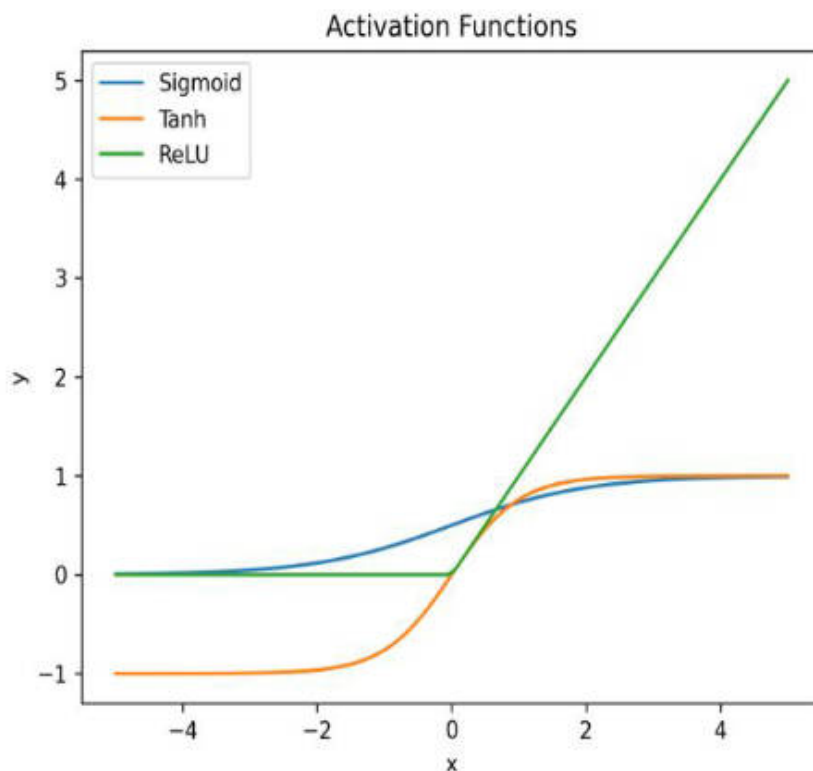
图 2.3 常用激活函数图像
