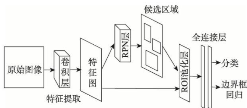
图 2.7 Faster R-CNN 模型结构图
