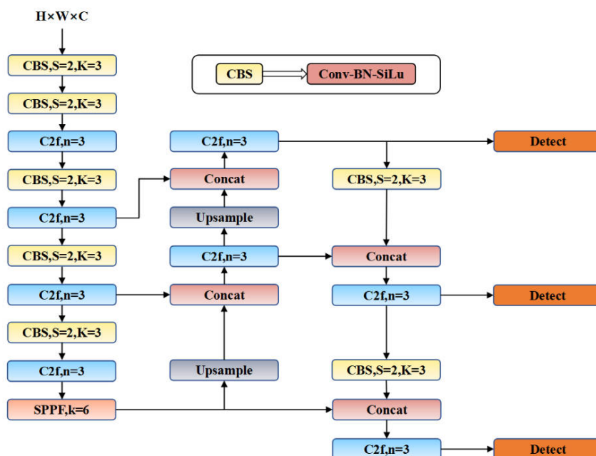
图 2.12 yolov8 整体框架图
