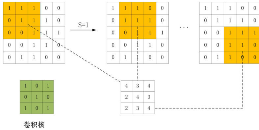
图 2-3 卷积运算过程
