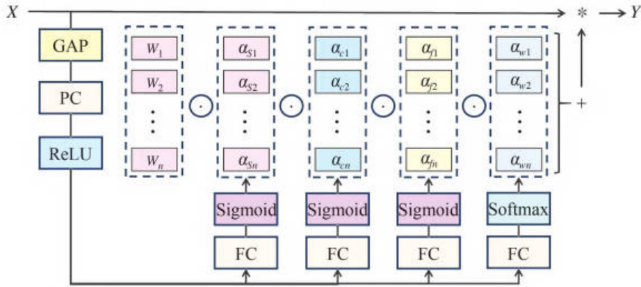
图 4.1 全维度动态卷积（待修改成横向的结构）
