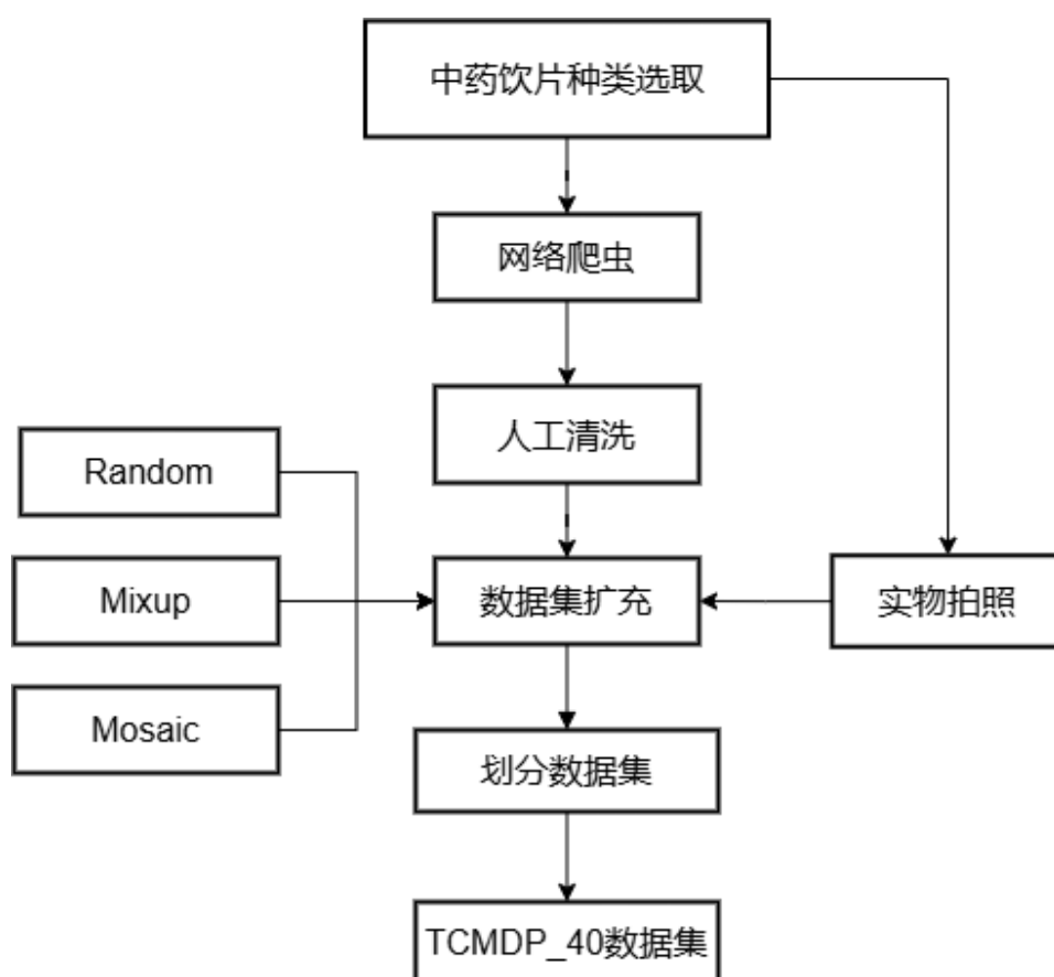
图 3.1 数据集构建流程图
