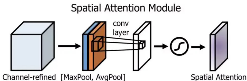
图 2.5 空间注意力
