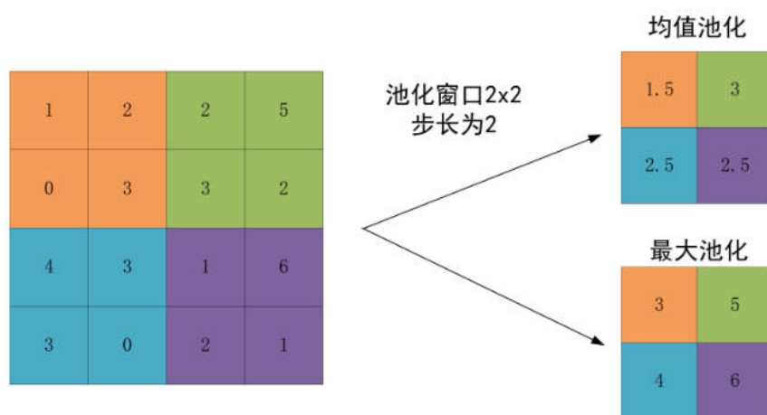
图 2-4 池化操作
