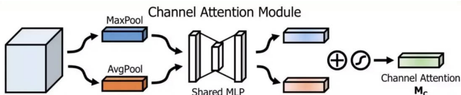
图 2.4 通道注意力模块
