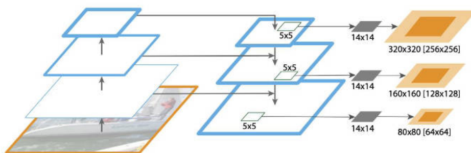
图 2.11 FPN 网络结构
