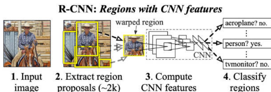
图 2.6 RCNN 模型结构
